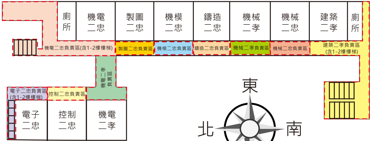
二樓平面圖
