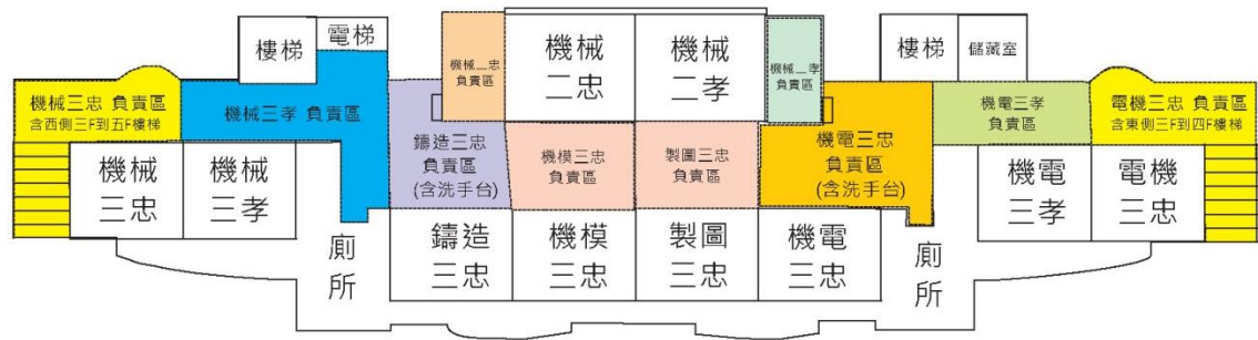
四樓平面圖
