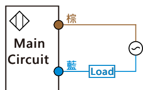
交流2線 NO/NC
