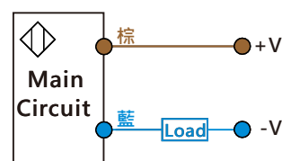
直流2線 PNP NO
